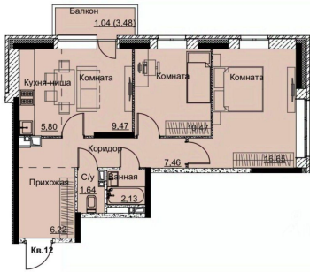
План 2 этажа Жилой дом №2
